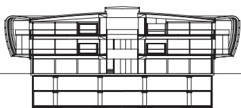
Coupe transversale
