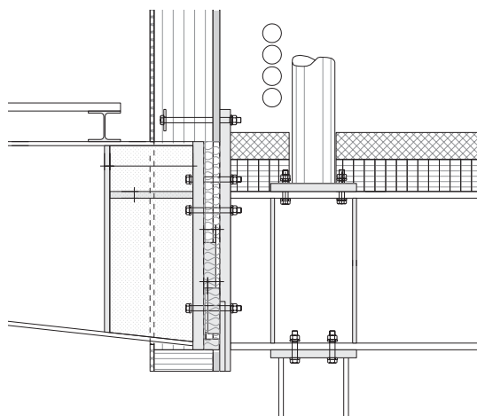
Detail plancher à l'étage, M 1:20
