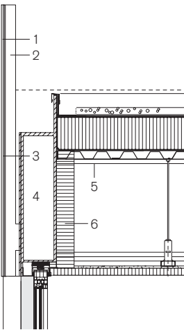
Détail foyer latéral, M 1:30
