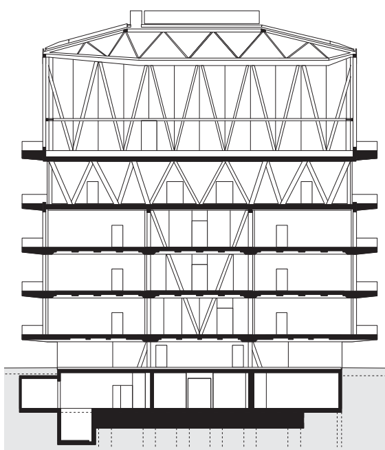
Coupe transversale
