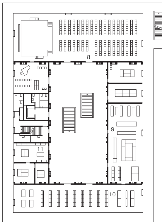
Plan du 4 e étage
