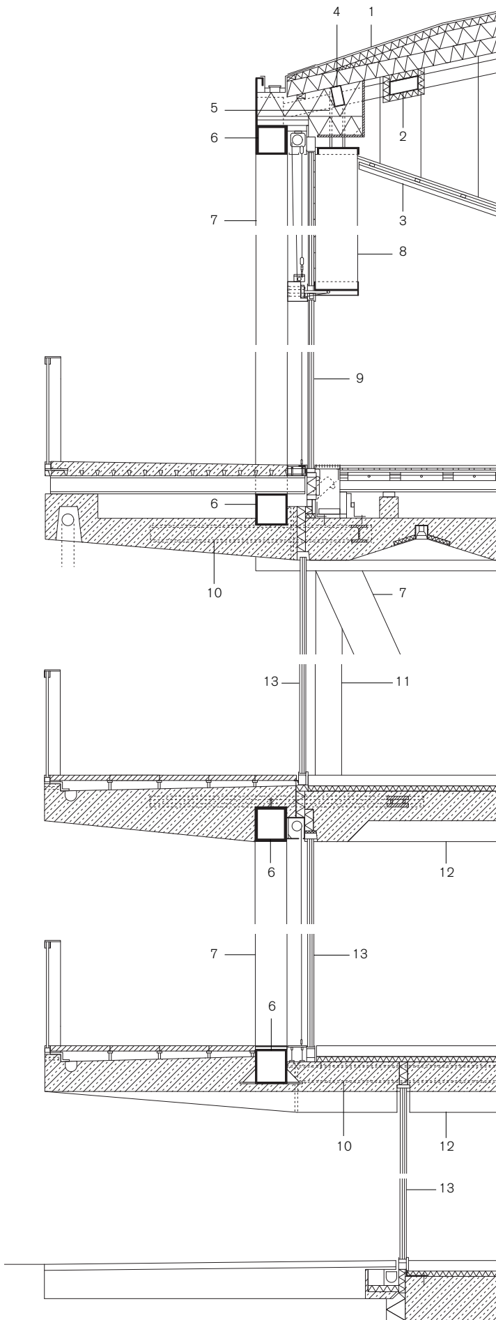
Coupe de façade, échelle 1:50
