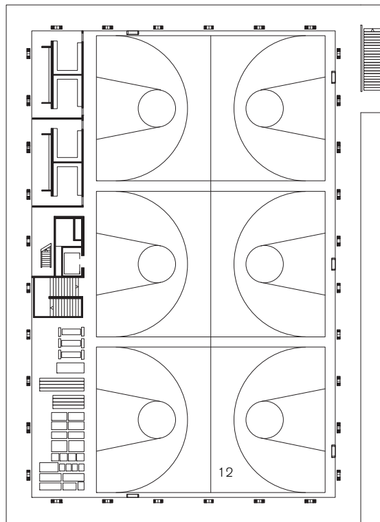
Plan du 5 e étage
