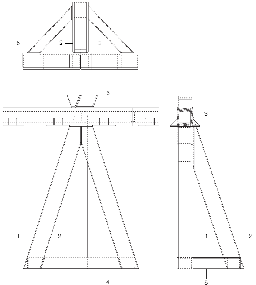
Poteau du rez-de-chaussée, échelle 1:50
