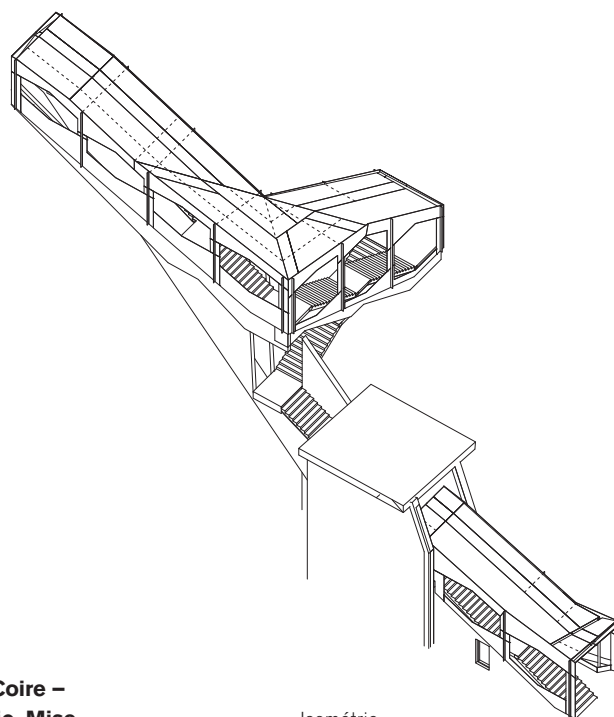
Isométrie
