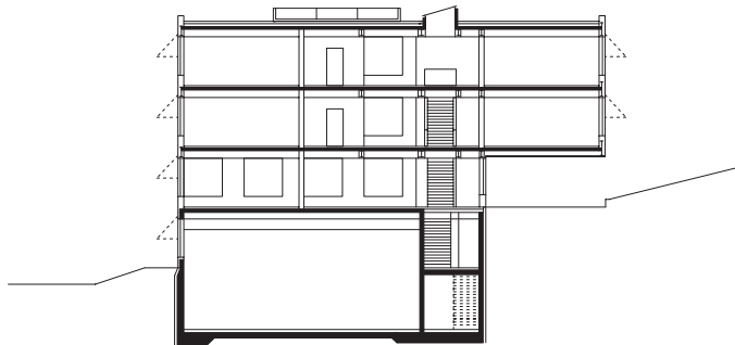
Querschnitt
