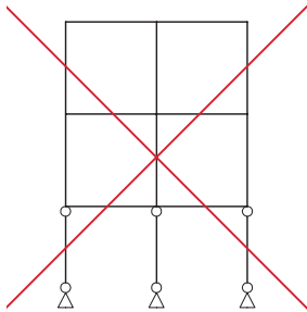
Falscher plastischer Mechanismus für duktiles Verhalten
